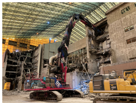
工場棟解体状況（東側）
