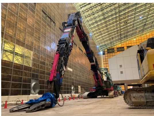
解体重機SK2200組立状況（東側）
