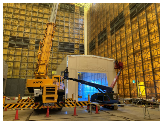
テント前室組立状況（北東側）
