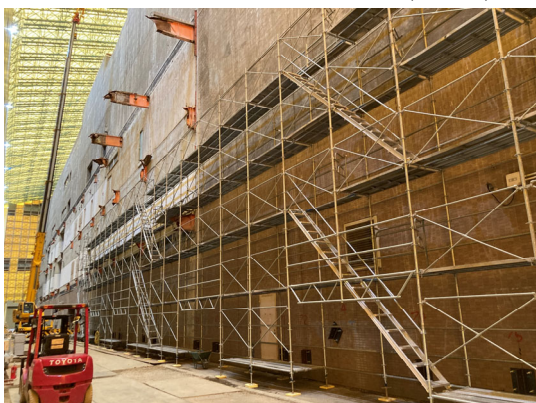
外壁撤去用足場組立状況（工場棟西側）
