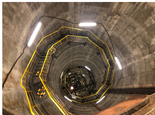
煙突内筒解体状況（地上50m）
