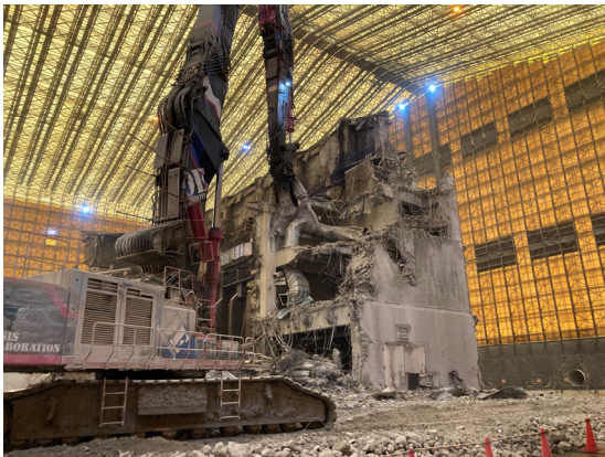
工場棟解体状況（北側）
