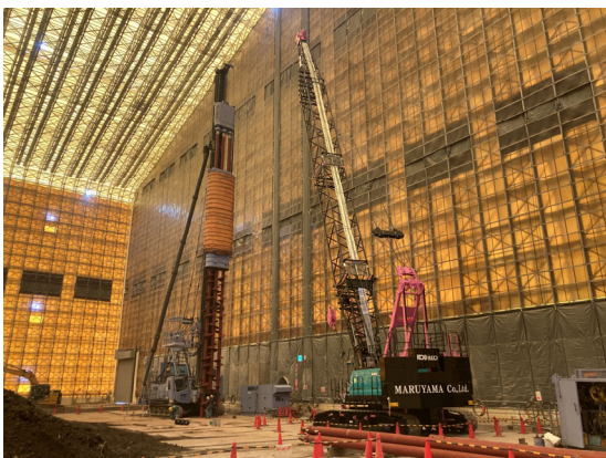
SMW工事重機組立状況（北側）
