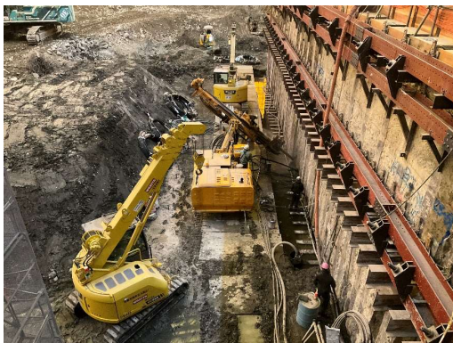
地盤アンカー施工状況（西側）
