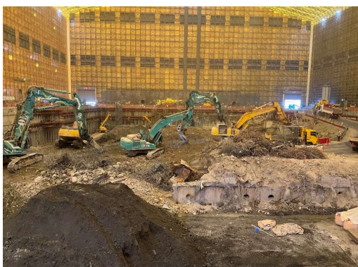
工場棟地下解体工事全景（南側）
