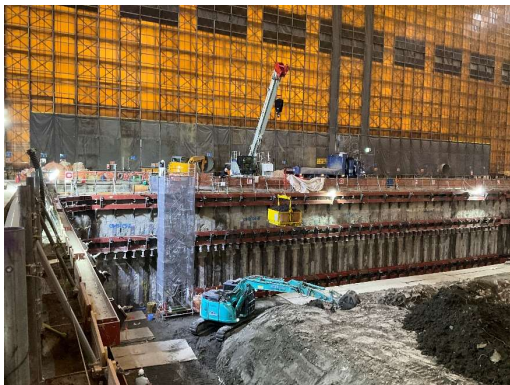
工場棟掘削工事施工状況（北側）
