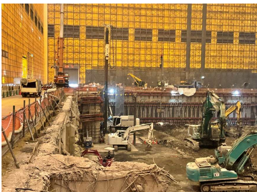
工場棟構台杭工事施工状況（西側）
