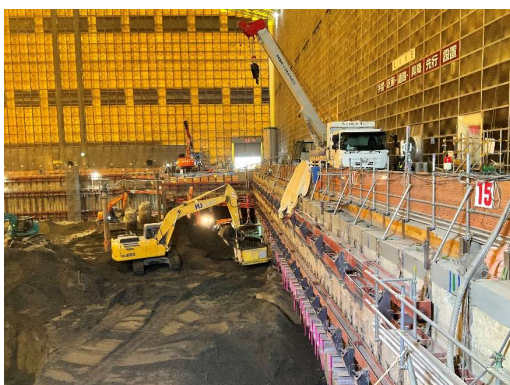
工場棟掘削状況（東側）
