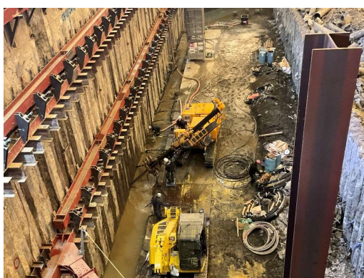
工事棟地盤アンカー施工状況（北側）
