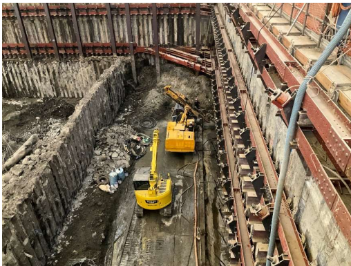
地盤アンカー打設状況（北側）
