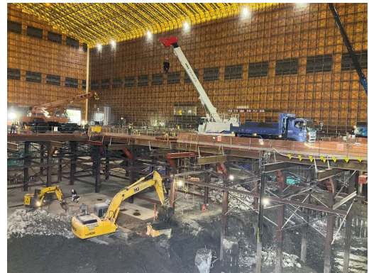
掘削残土積込み状況（南側）
