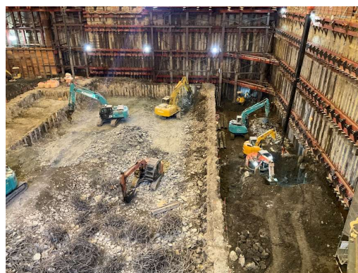
掘削解体施工状況（北側）
