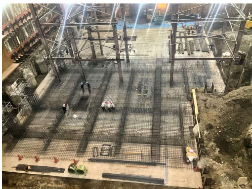
地下2階基礎配筋状況（南側）
