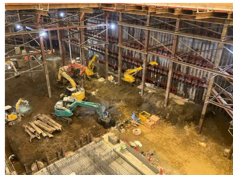
掘削状況（東側）
