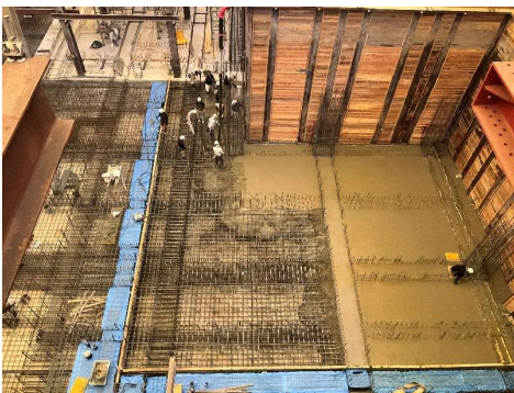
コンクリート打設状況（西側）
