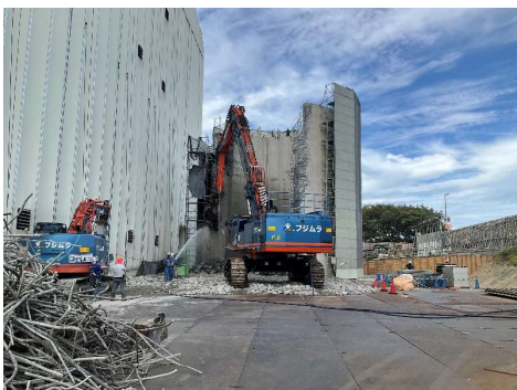
煙突外筒解体施工状況
