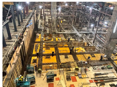
ピット階躯体工事施工状況（西側）
