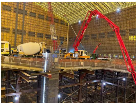
工場棟全覆いテント内コンクリート打設状況①（中央部）
