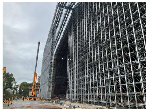
全覆いテント妻面盛替施工状況（南側）
