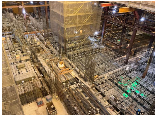
工場棟地下2階施工状況（中央部）
