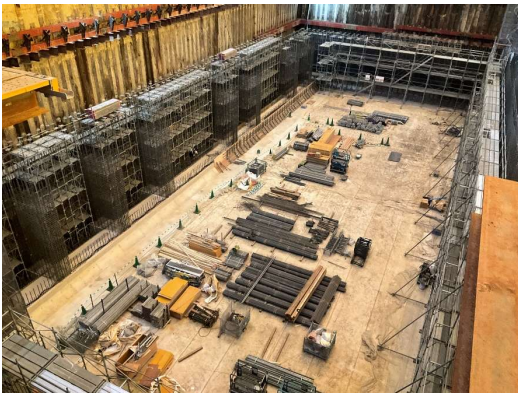
工場棟地下2階施工状況（北側）
