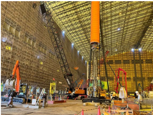
工場棟既製杭打設状況（西側）
