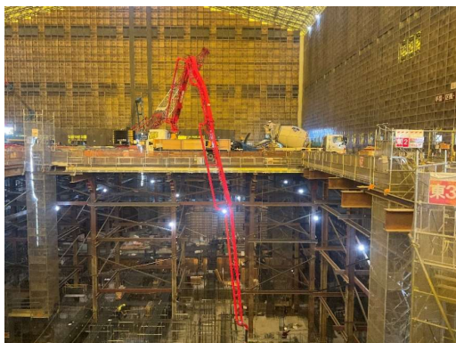
工場棟地下2階躯体工事コンクリート打設状況（東側）
