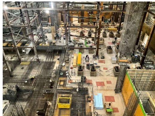
工場棟地下2階躯体工事施工状況（中央部）
