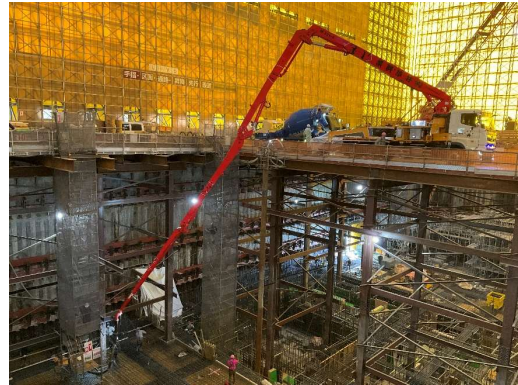
工場棟地下2階躯体工事施工状況コンクリート打設（中央部）
