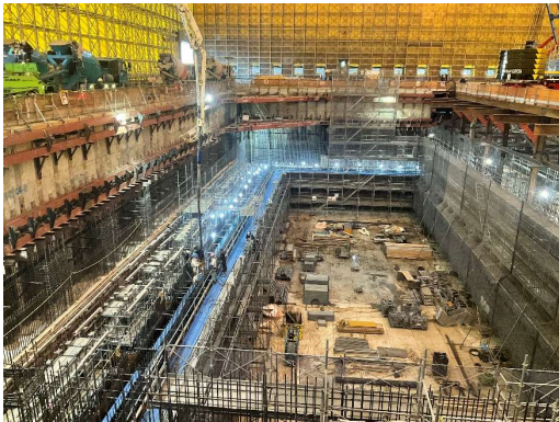
工場棟ごみバンカ地下2階躯体施工状況（北側）
