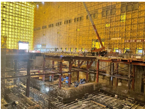
構台解体施工状況（西側）
