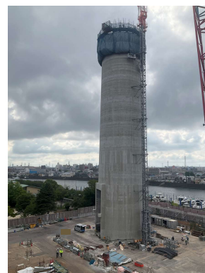
煙突地上躯体工事施工立状況
