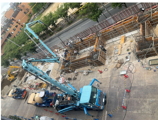
工場棟あと施工西工区基礎躯体工事コンクリート打設状況（北東側）
