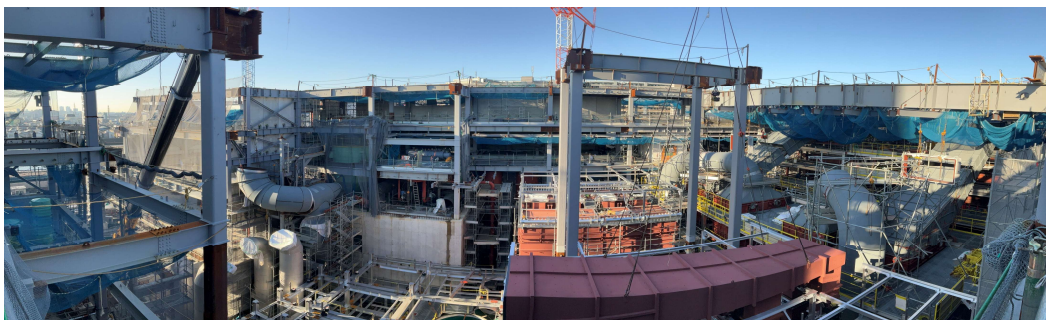
工場棟地上躯体工事施工状況（中央部）
