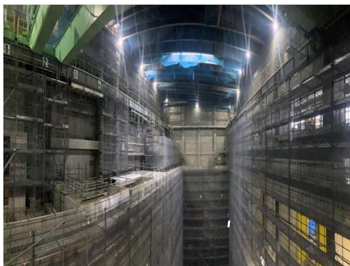
工場棟ごみバンカ地上躯体工事施工状況
